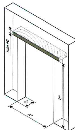
Конструкция внутри проема
