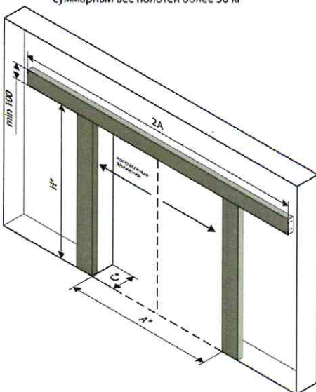
Фиксация усиления проема к стенам и перекрытиям
