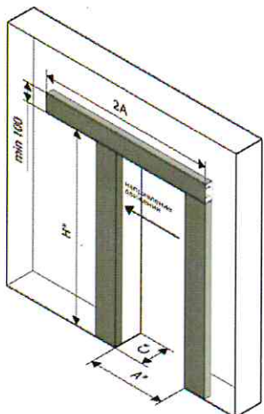
Однстворчатая конструкция вдоль проема вес полотна более 50 кг
